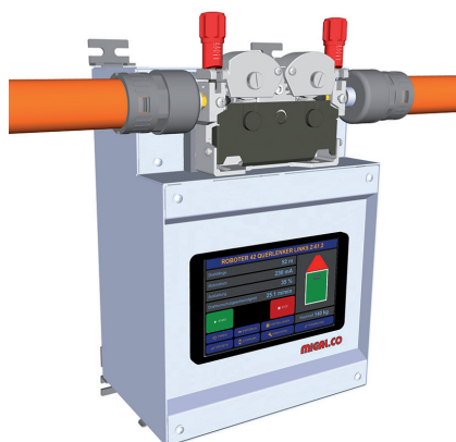
Bedienpanel um 90° gedreht für horizontale Drahtlaufichtung
