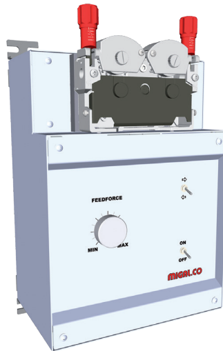
Bedienpanel um 90° gedreht für horizontale Drahtlaufrichtung
