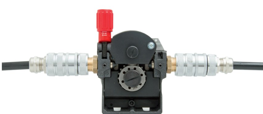
Druckluft-Drahtantrieb DLDA-1 mit Drahtführungsschlauch in Ein- und Ausgang
