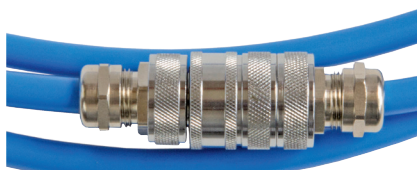
Softliner-Detail mit Kupplung CRNG40
