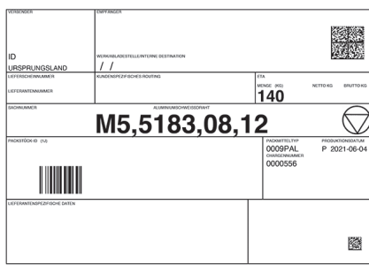
Datamatrix code (VDA-label) für Chargennummer, Gewicht, Produktionsdatum und Artikelnummer
