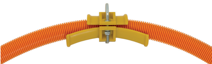
Schlauchhalterung für Rolliner NG, Rolliner 3G sowie für Schutzschlauch PA12
