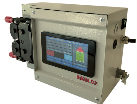
RoboFeed Wire Manager Seitenansicht
